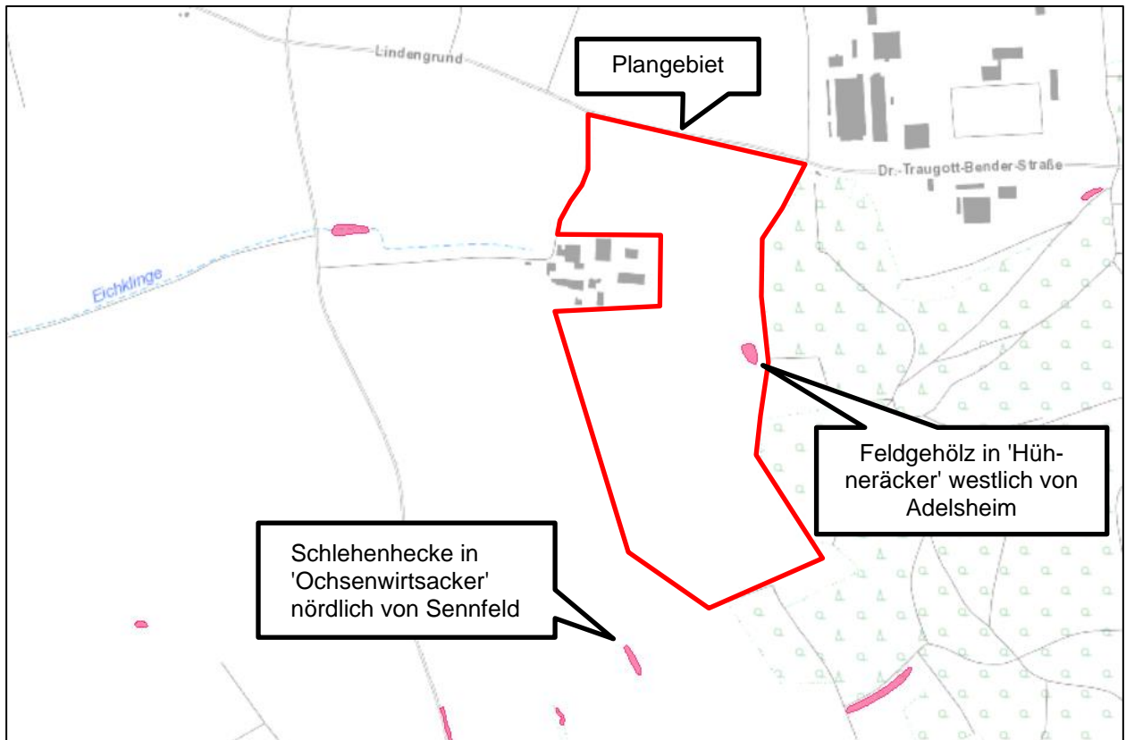
Abb. 9: gesetzlich geschützte Biotope; © Grundlage: Daten aus dem Umweltinformationssystem (UIS) der LUBW Landesanstalt für Umwelt Baden-Württemberg; Plangebiet grob markiert durch Enviro-Plan 2023
