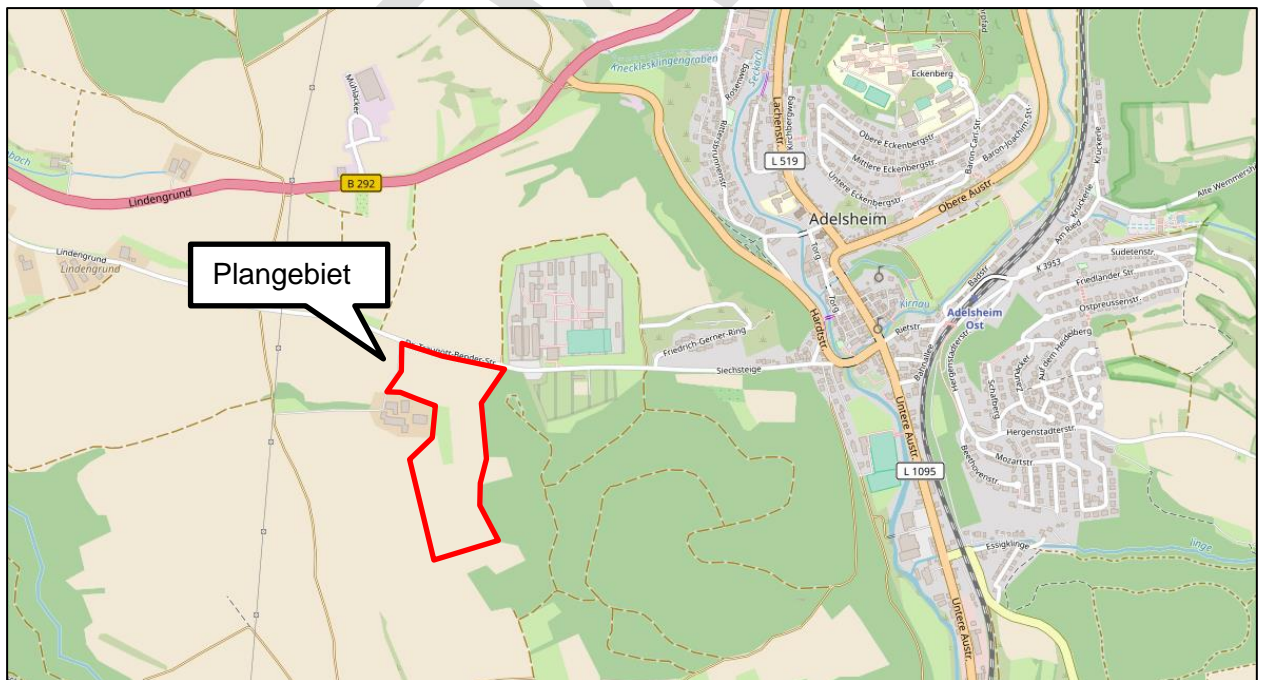
Abb. 2: Plangebiet; unmaßstäblich ©OpenStreetMap-Mitwirkende, www.openstreetmap.org/copyright ; Plangebiet ergänzt durch Enviro-Plan 2023
