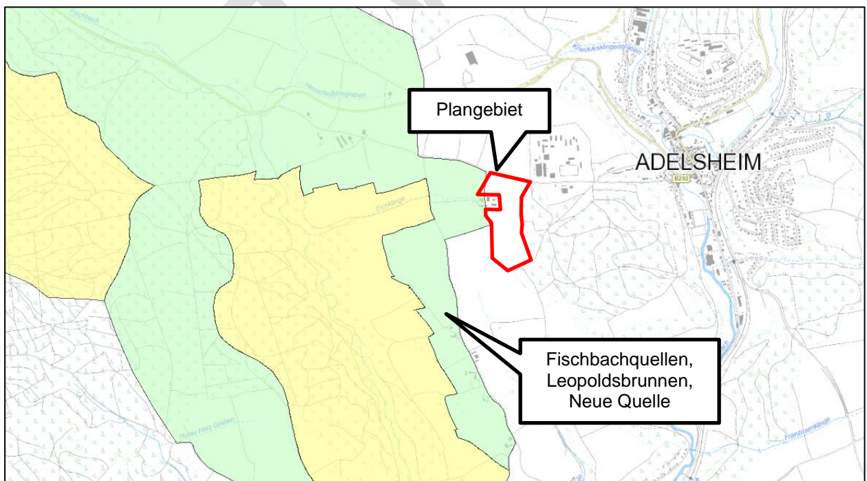
Abb. 10: Wasserschutzgebietszonen; © Grundlage: Daten aus dem Umweltinformationssystem (UIS) der LUBW Landesanstalt für Umwelt Baden-Württemberg; Plangebiet grob markiert durch Enviro-Plan 2023
